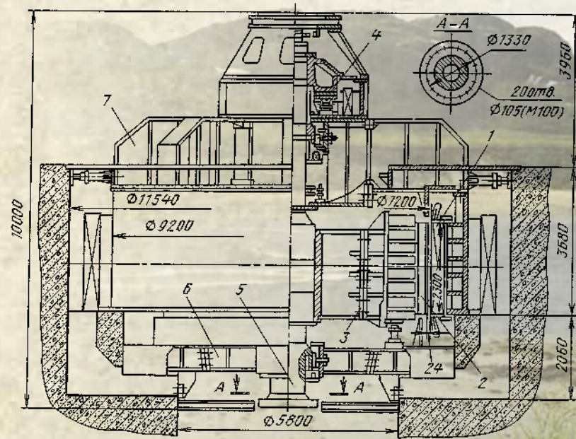
Рис.18.3. Гидрогенератор Верхне-Териберской ГЭС ( N = 130 МВт; u = 10,5 кВ; n = 187,5 об/мин): 1 — сердечник статора; 2 — полюсы; 3 — осто́в ротора; 4 — подпятники; 5 — вал ротора; 6 — нижняя крестовина; 7 — верхняя крестовина
